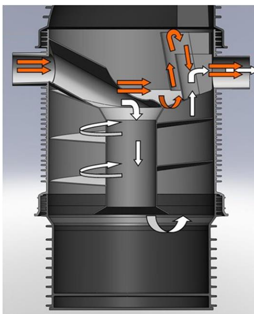
Рис. 1 Принцип работы отделителя
