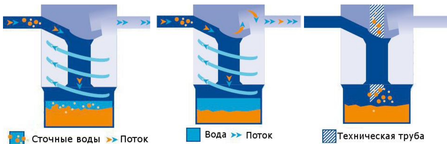
Рис. 1 Принцип работы отделителя
