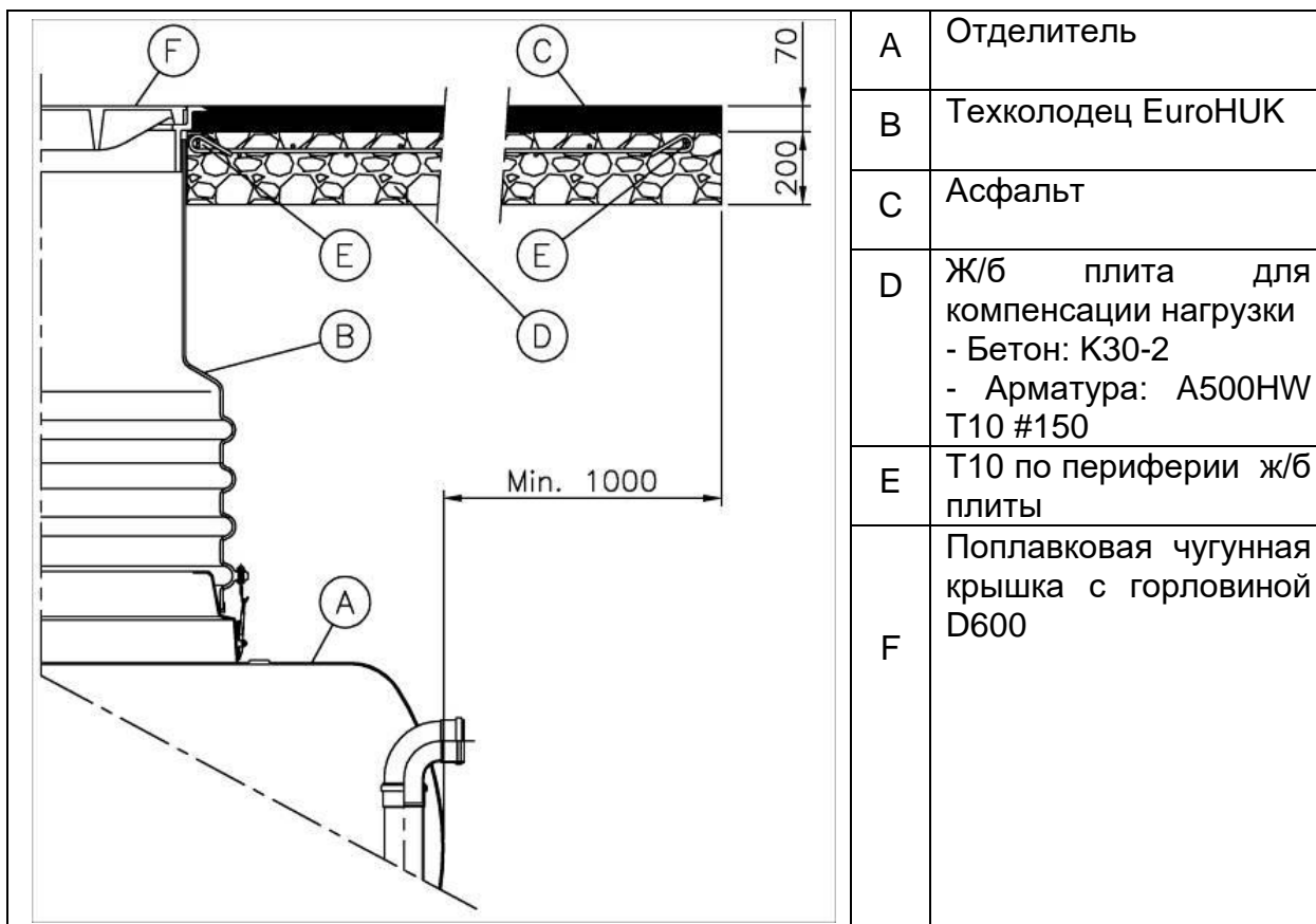
Рис. 7. Конструкция несущей плиты.
