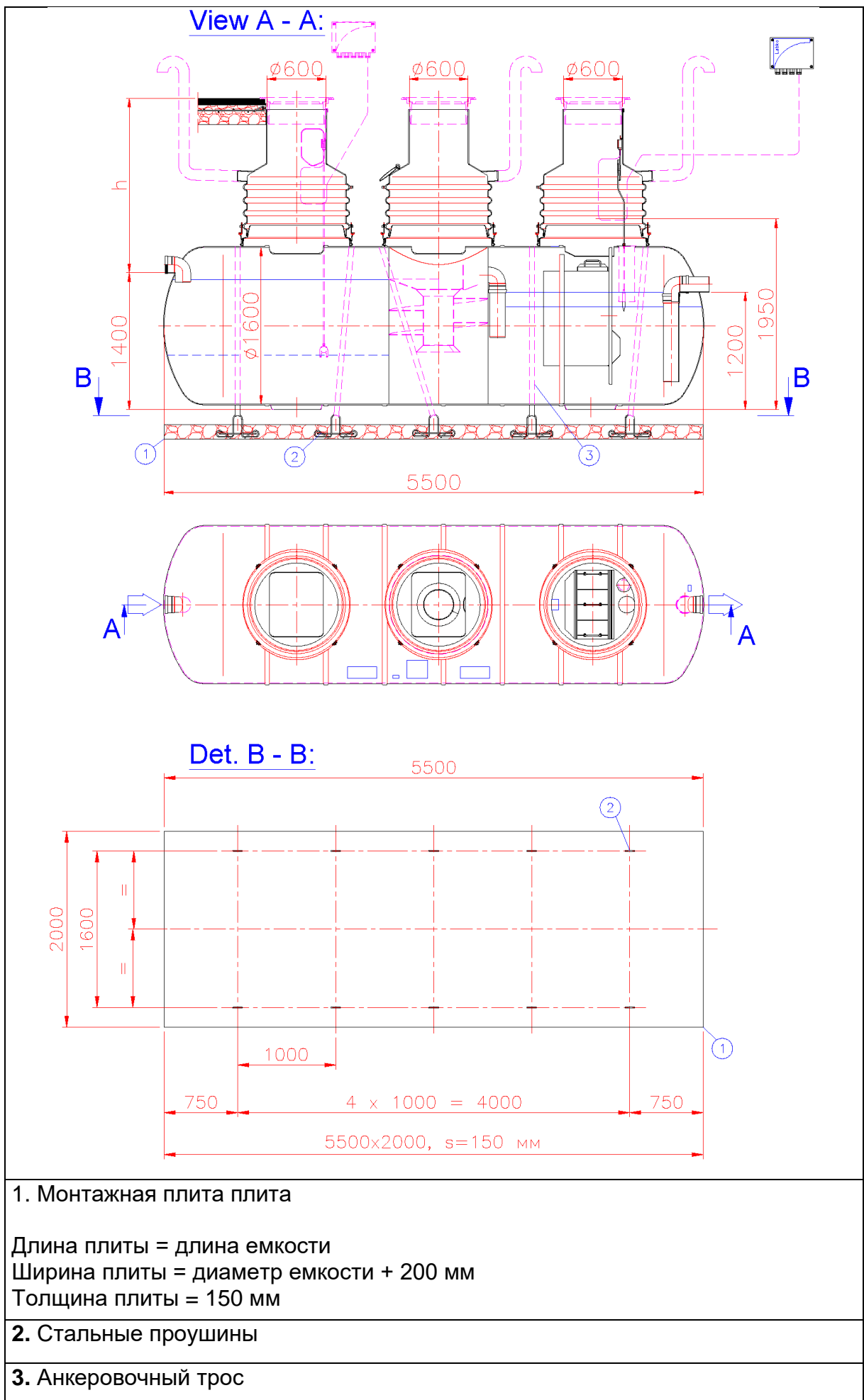
Рис. 4. Крепление корпуса при высоком уровне грунтовых вод или при слабо несущем грунте.
