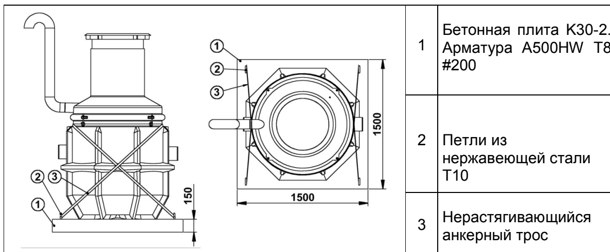
Рис. 3. Анкерка нефтемаслоотделителя (при необходимости).
