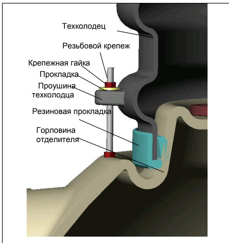
Рис 3. Крепление техколодца EuroHUK к отделителю EuroHEK Omega.
